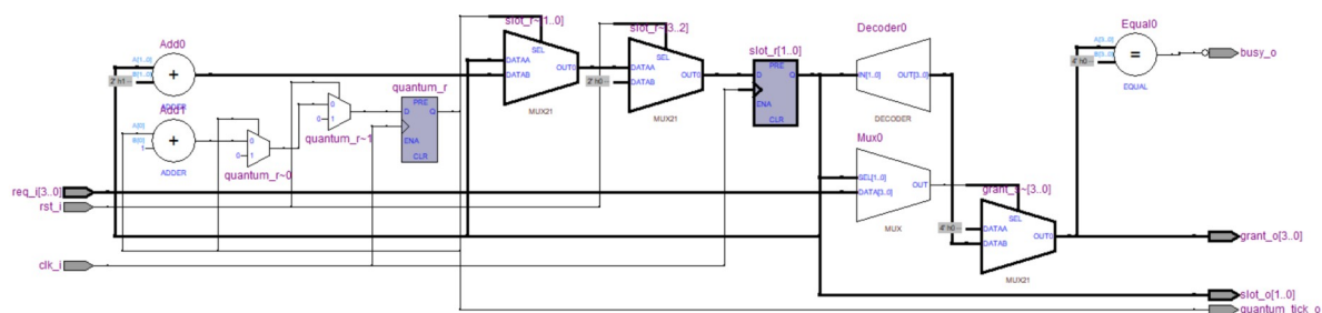
Рисунок 4.4 – Схема центрального арбитра с фиксированным временным квантом
