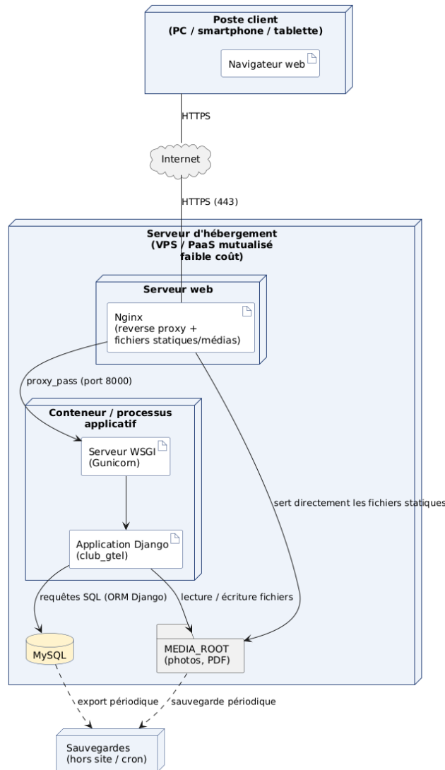
Figure 8 — Diagramme de déploiement
