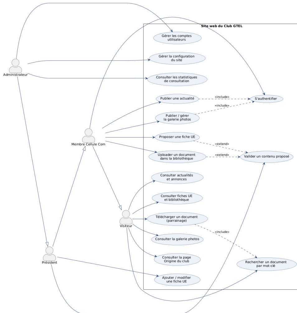
Figure 1 — Diagramme de cas d'utilisation du site du Club GTEL
