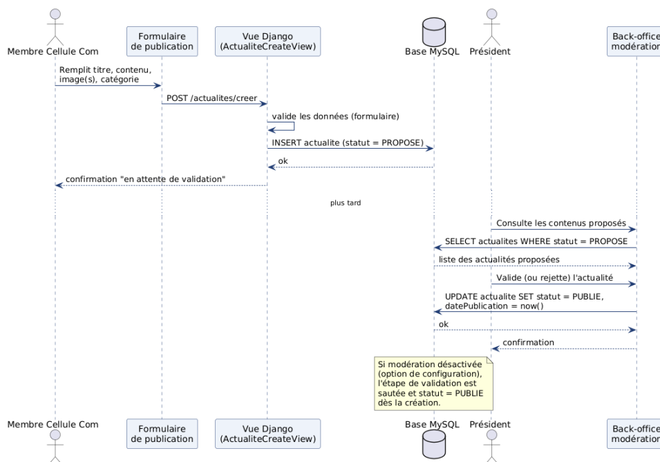
Figure 4 — Séquence : publication et validation d'une actualité
