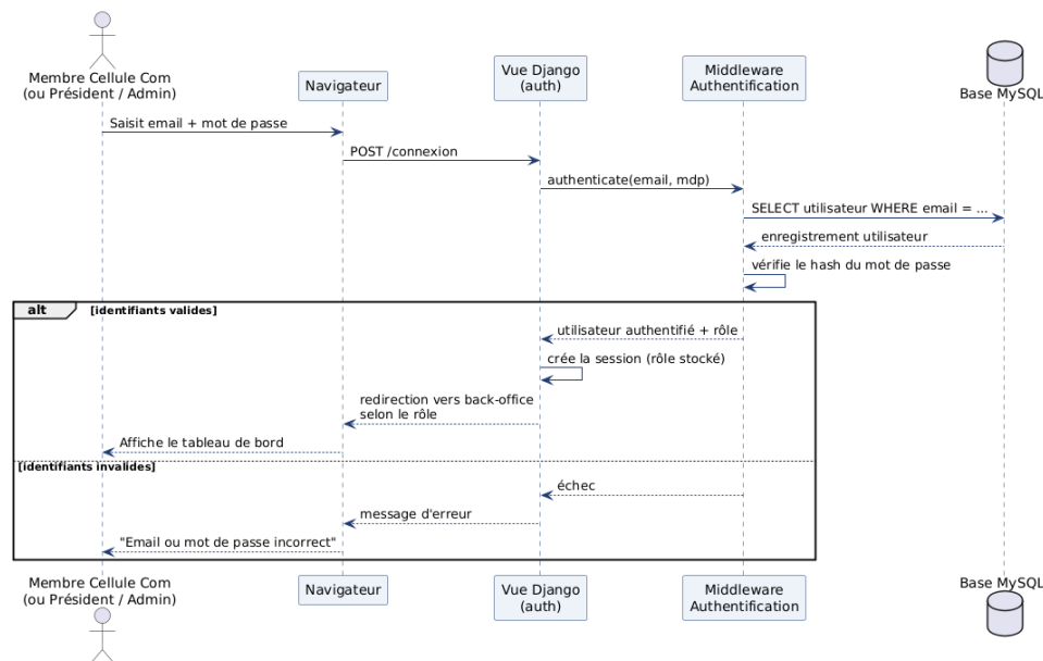
Figure 3 — Séquence : authentification
