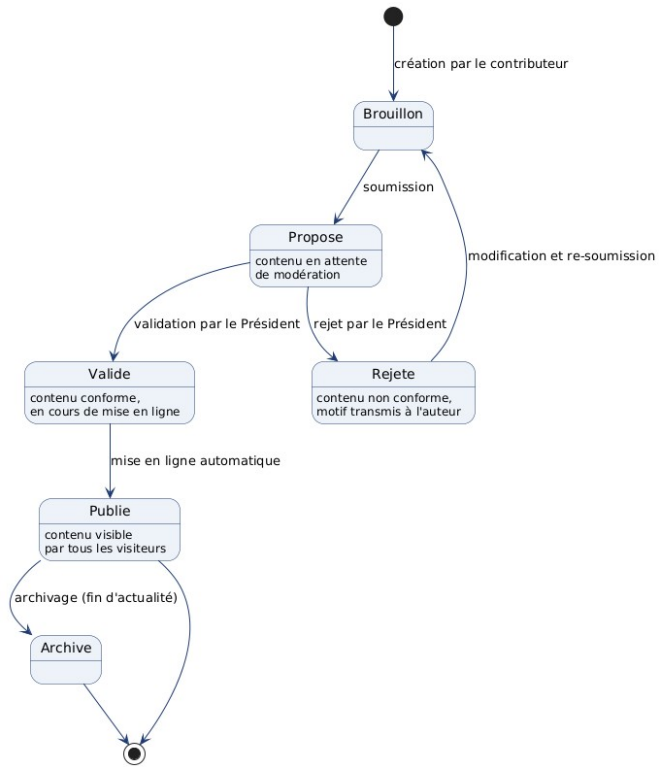
Figure 7 — Diagramme d'état-transition du statut d'un contenu
