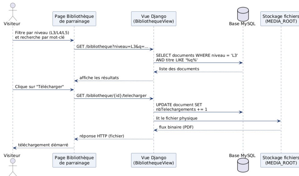
Figure 5 — Séquence : recherche et téléchargement d'un document de la bibliothèque
