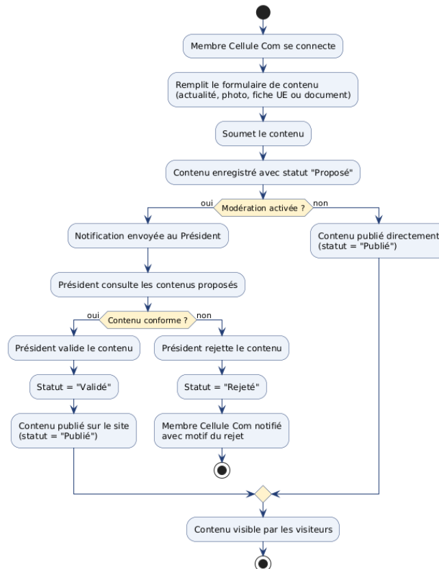
Figure 6 — Diagramme d'activité : workflow de publication d'un contenu
