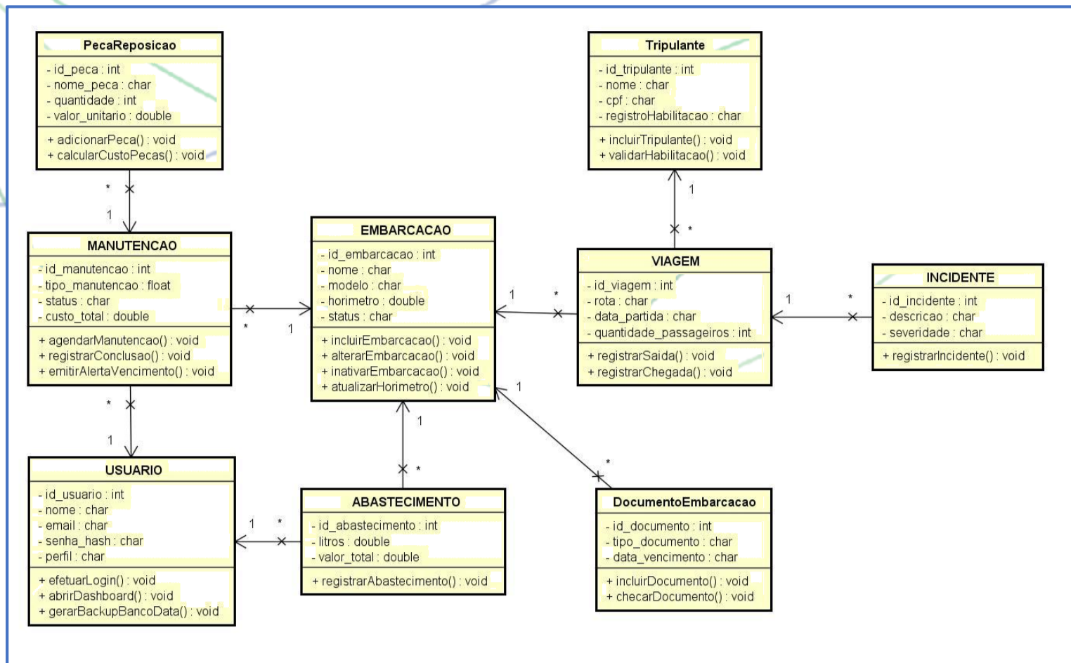
Diagrama de Classes do Sistema
