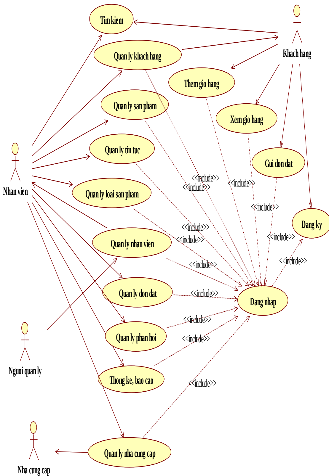
Hình 6. Mô hình Use - Case
