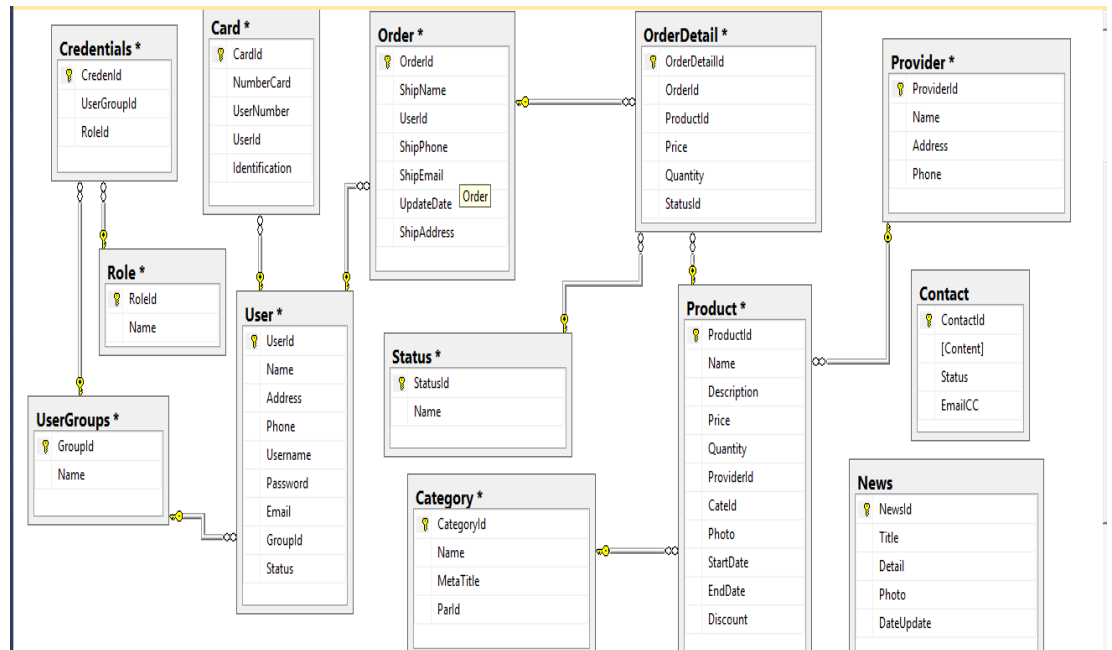
Hình 16. Sơ đồ Diagram
