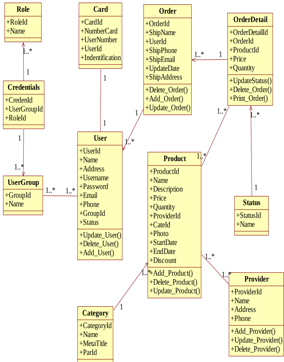
Hình 15. Biểu đồ lớp chi tiết
