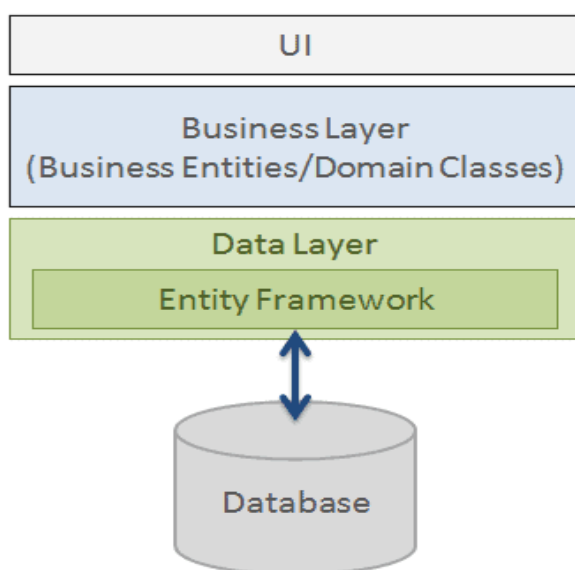
Hình 2. Entity Framework
