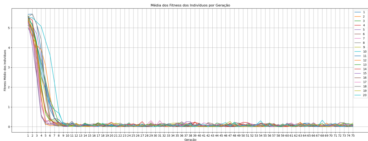
Figura 2: Comportamento do fitness médio dos indivíduos em 20 execuções diferentes para o mesmo conjunto de parâmetros
