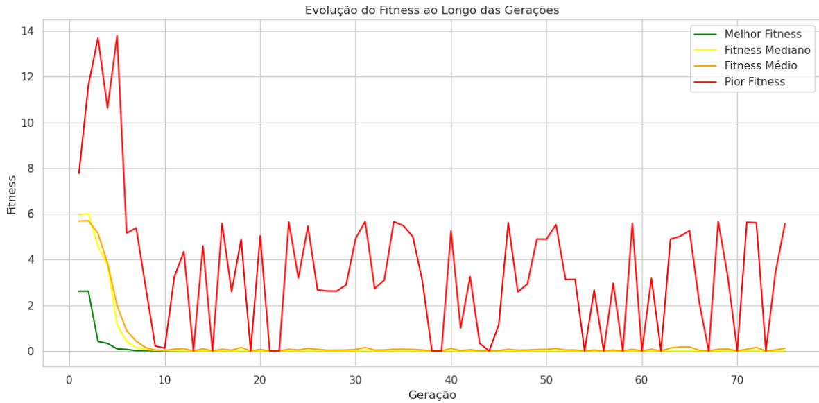
Figura 1: Comportamento dos valores de fitness dos indivíduos ao longo da execução
