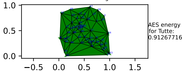
Tutte Embedding
