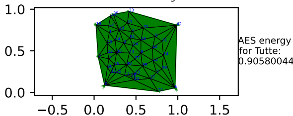
Tutte Embedding
