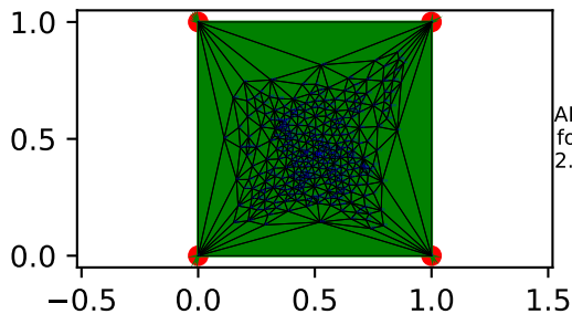
Tutte Embedding
