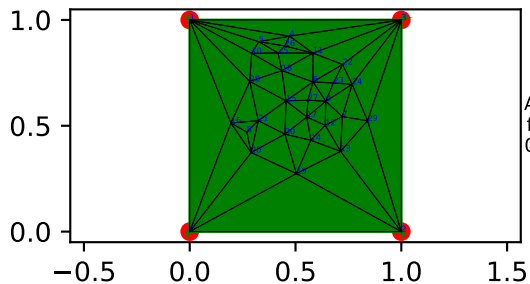
Tutte Embedding
