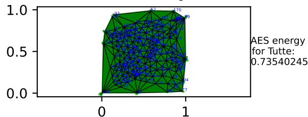
Tutte Embedding
