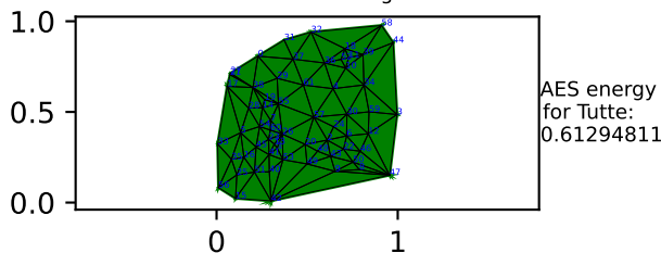
Tutte Embedding
