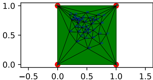
Tutte Embedding
