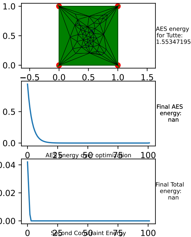
Tutte Embedding
