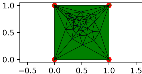
Tutte Embedding
