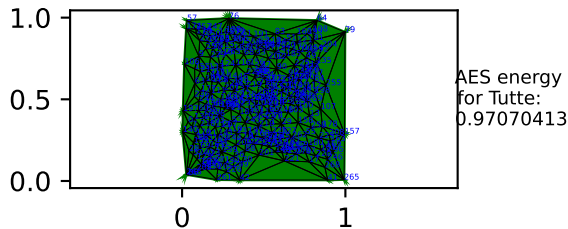
Tutte Embedding
