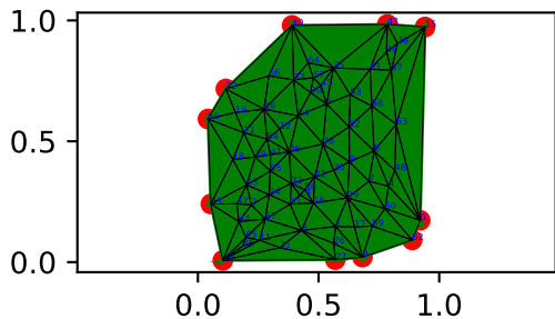
Tutte Embedding
