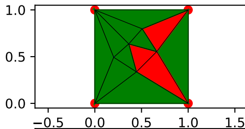
Tutte Embedding
