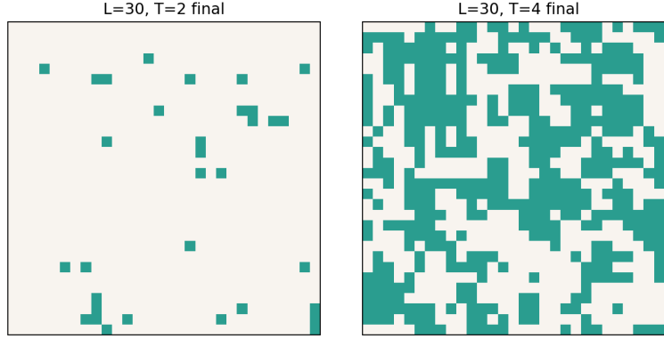
图 7: 二维 Ising 在 T=2 和 T=4 的最终自旋图样
