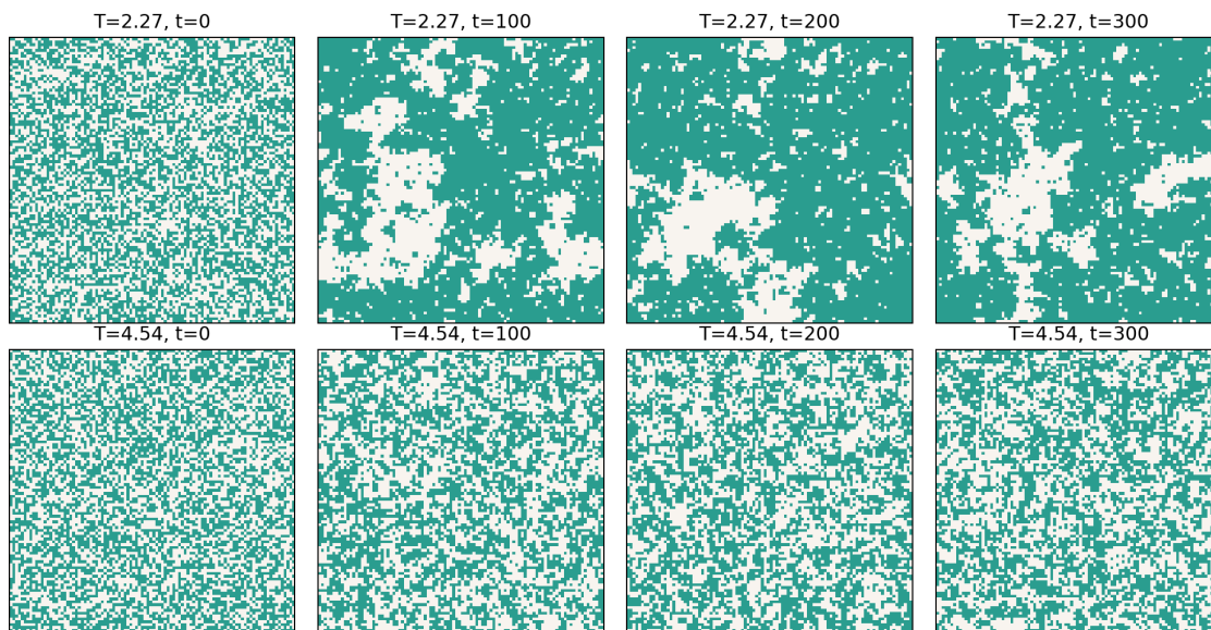
图 15: 100x100 二维 Ising 自旋图样演化
