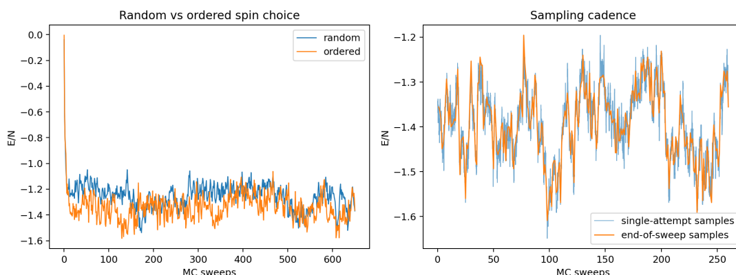
图 12: 更新顺序与采样间隔比较
