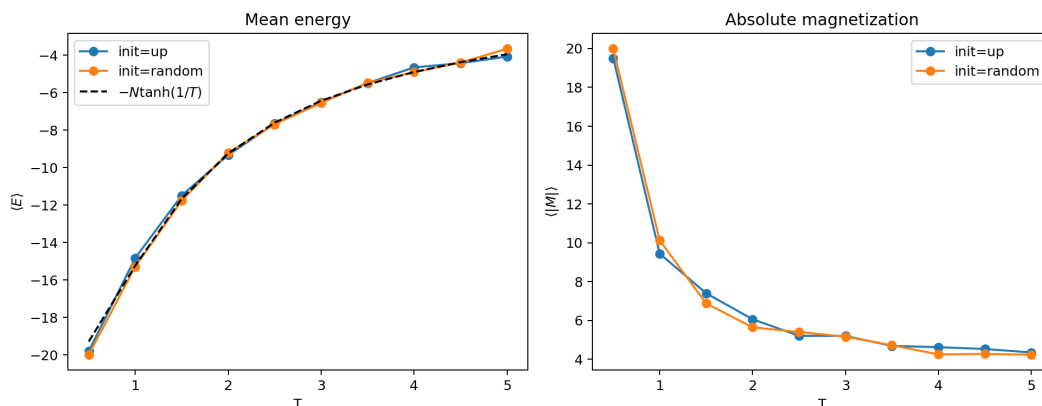
图 2: 一维 Ising 链的温度扫描
