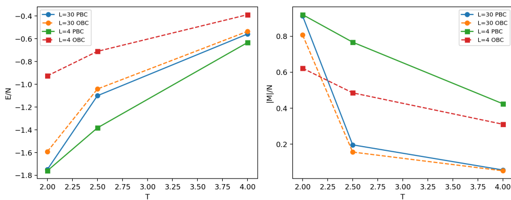
图 11: 开放边界与周期边界比较
