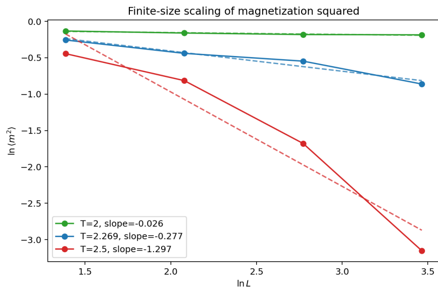
图 14: 磁化平方的有限尺寸标度拟合
