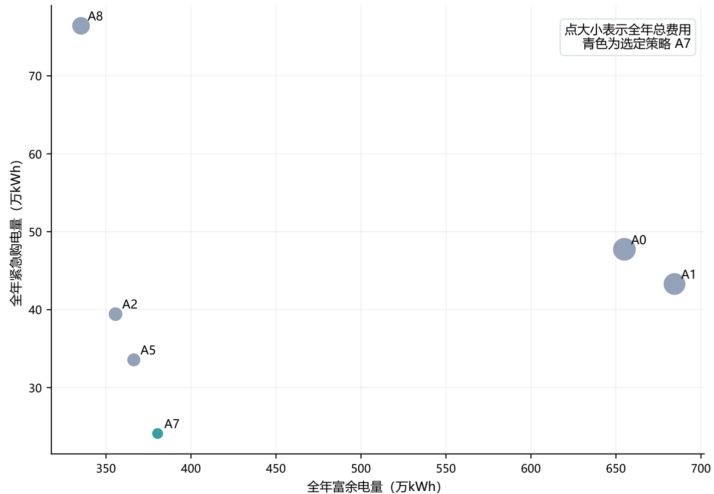
问题2：代表性策略的富余—紧急购电权衡
