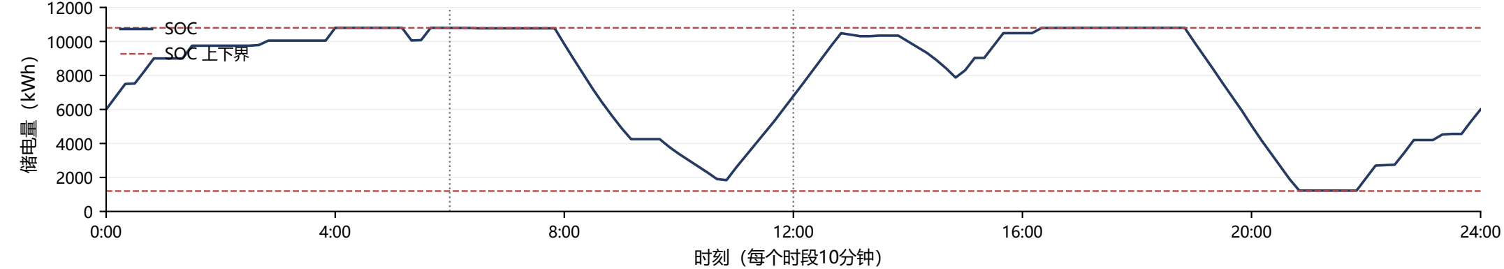
储能荷电状态
