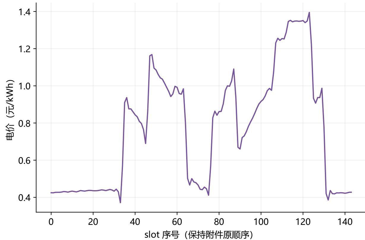
日电价曲线
