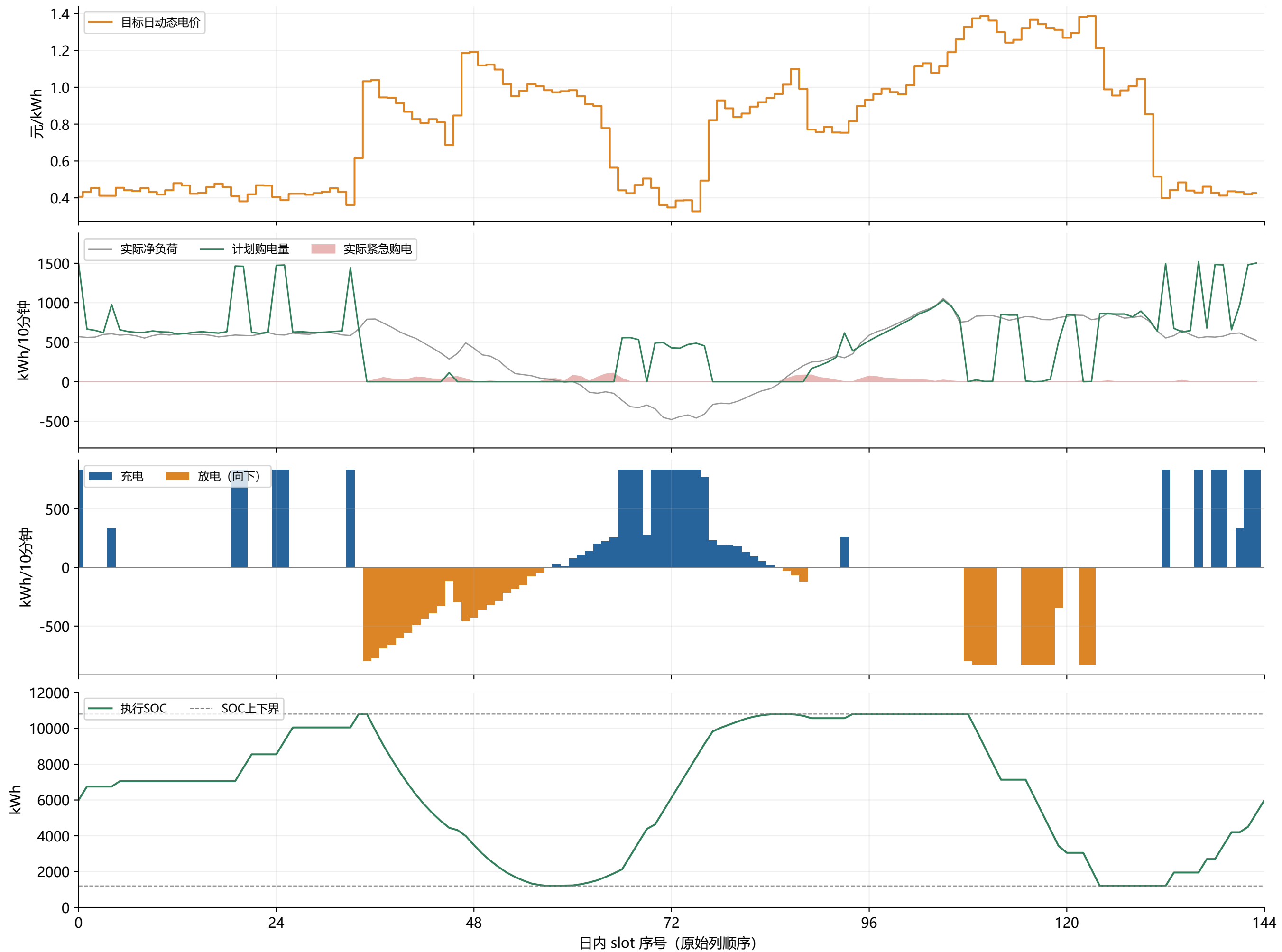
问题4-2 | 2025-09-23 调度与结算 全天总费用 52,010.63 元
