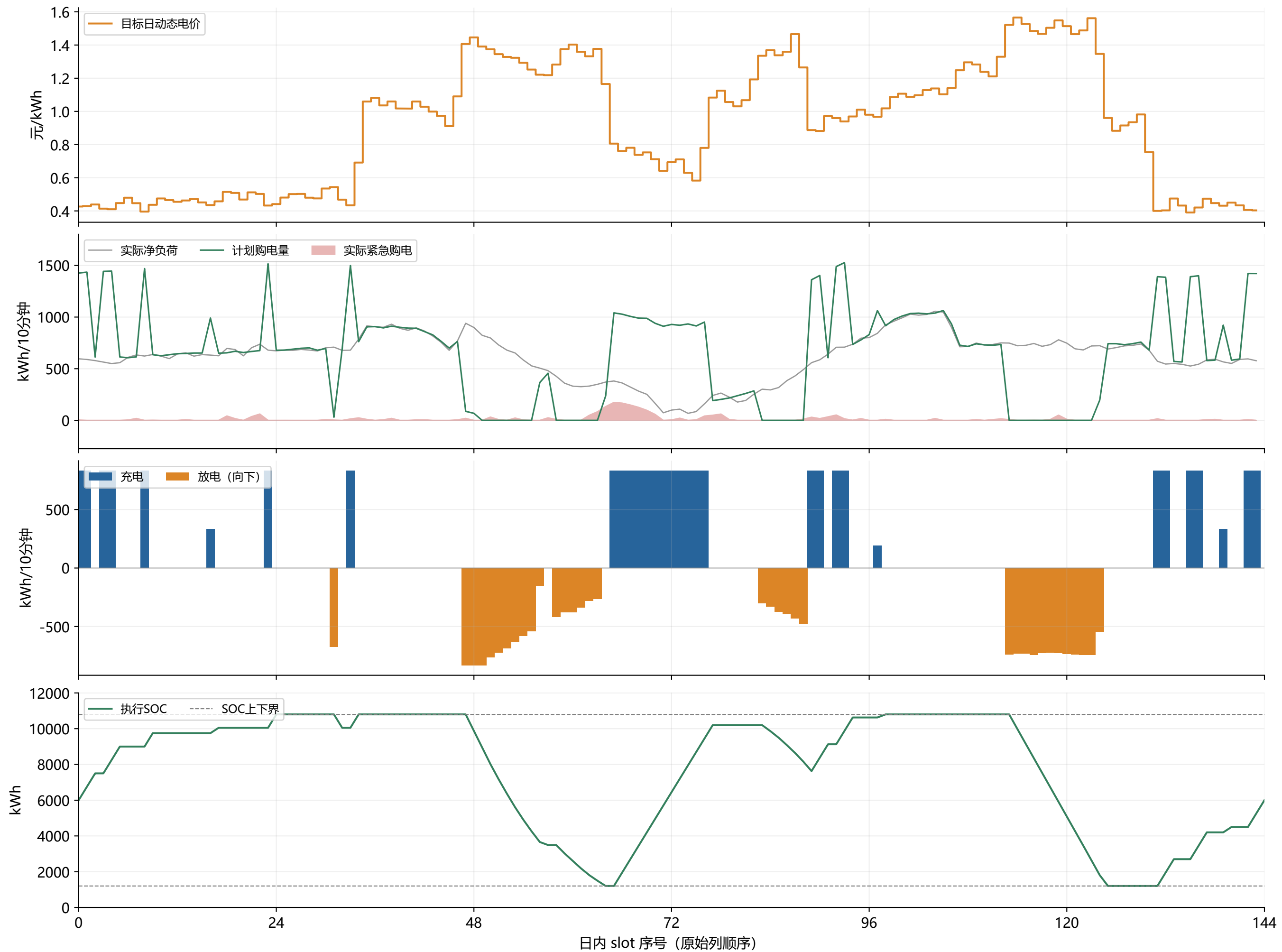
问题4-2 | 2025-12-21 调度与结算 全天总费用 78,423.13 元
