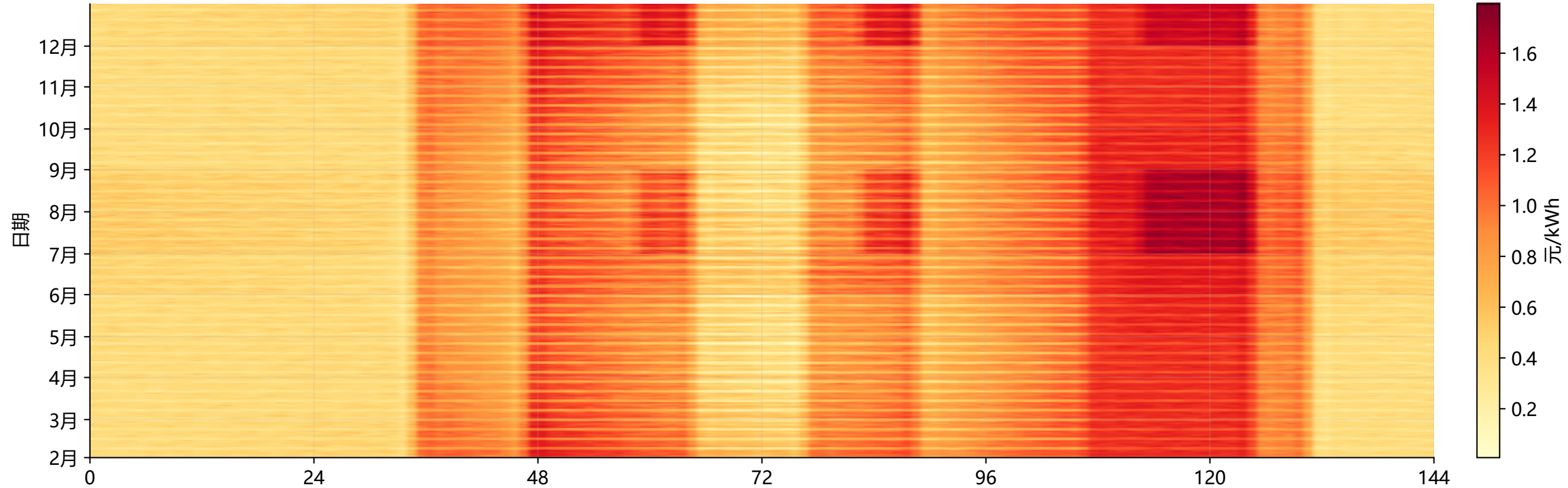
问题4-3 | 动态电价分布 (2025年2—12月) 每日144点结算电价
