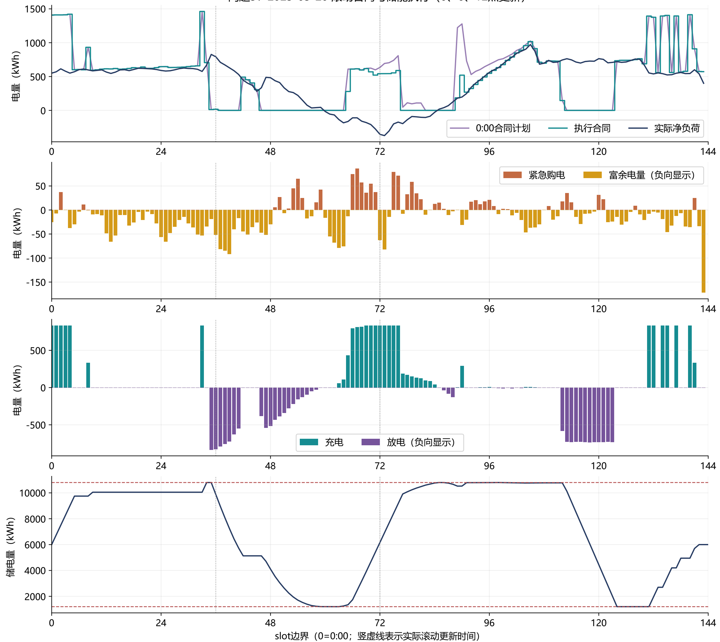
问题3：2025-03-20 滚动合同与储能执行 (0、6、12点更新)
