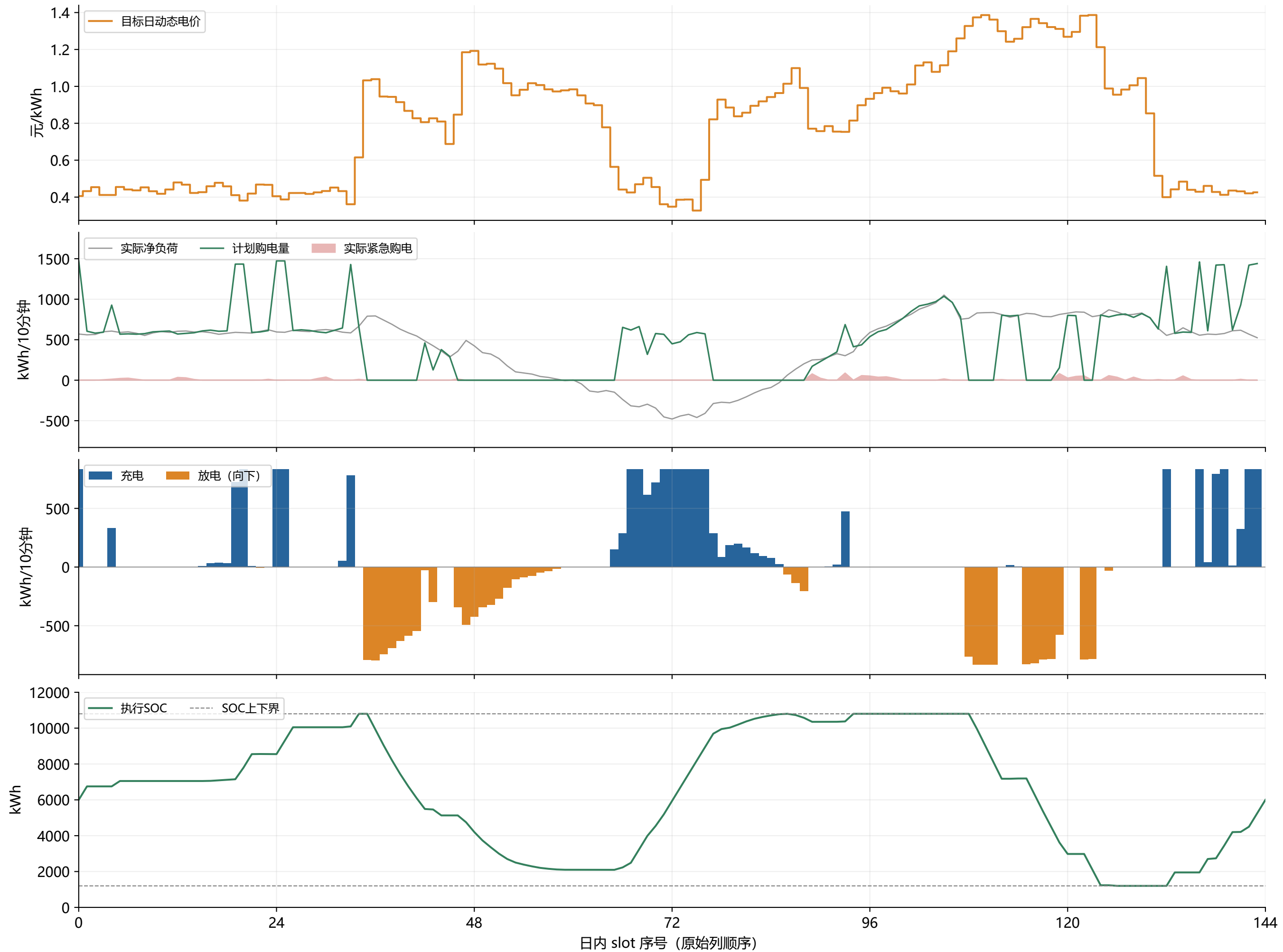
问题4-2 | 2025-09-23 调度与结算 全天总费用 48,568.84 元
