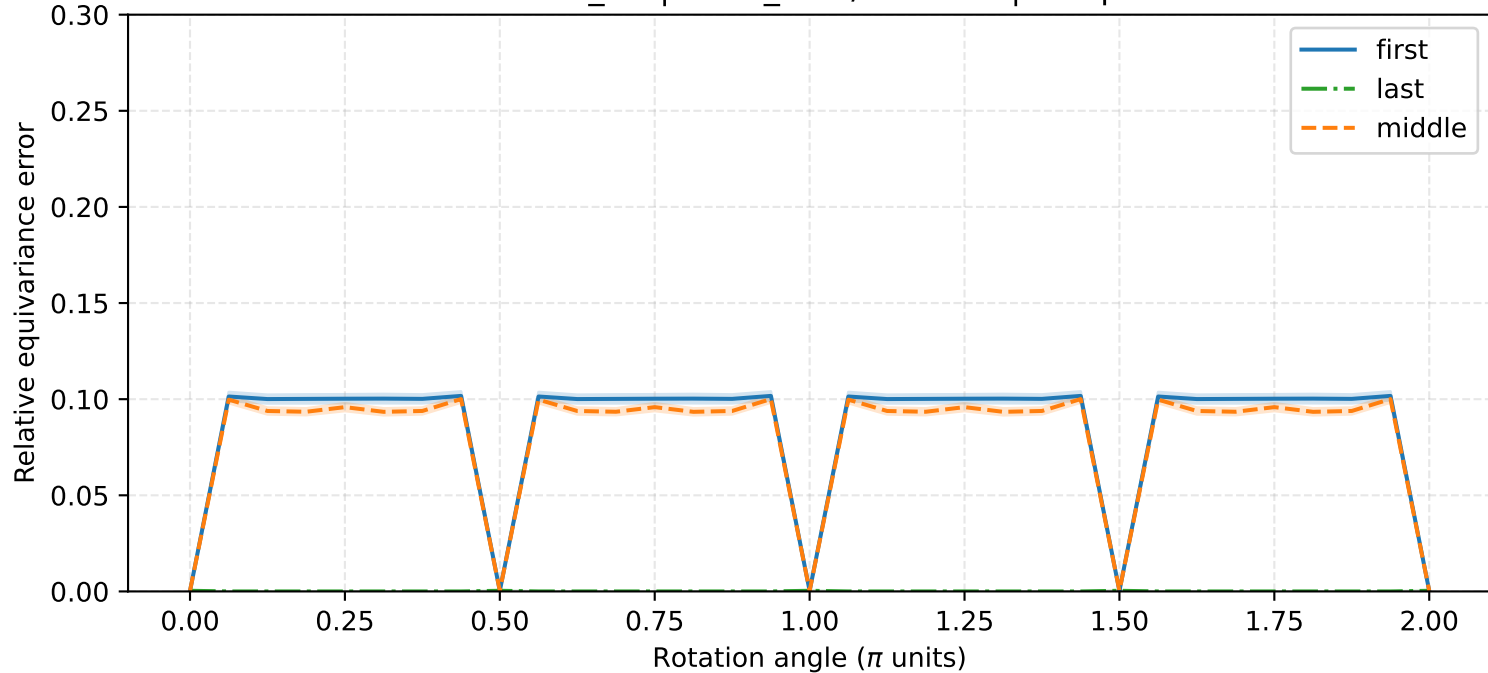
mnist_rot | norm_relu / Normbn | noflip
