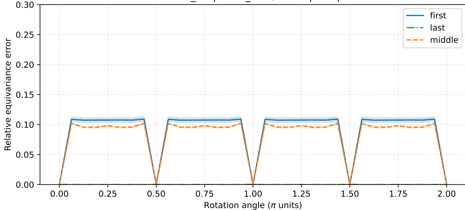
mnist_rot | norm_relu / IIDbn | noflip
