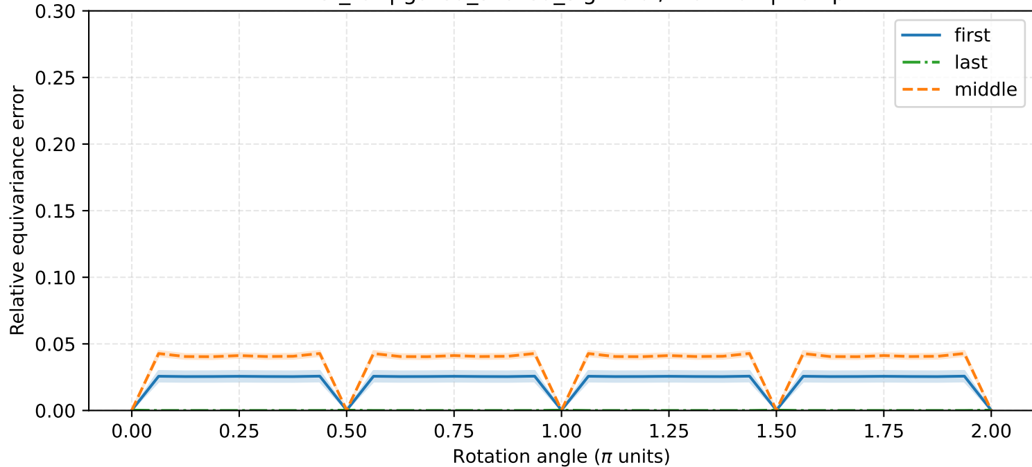
mnist_rot | gated_shared_sigmoid / Normbn | noflip
