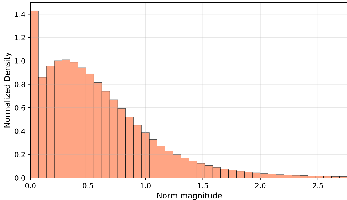
fourierbn_relu_16 + Normbn
