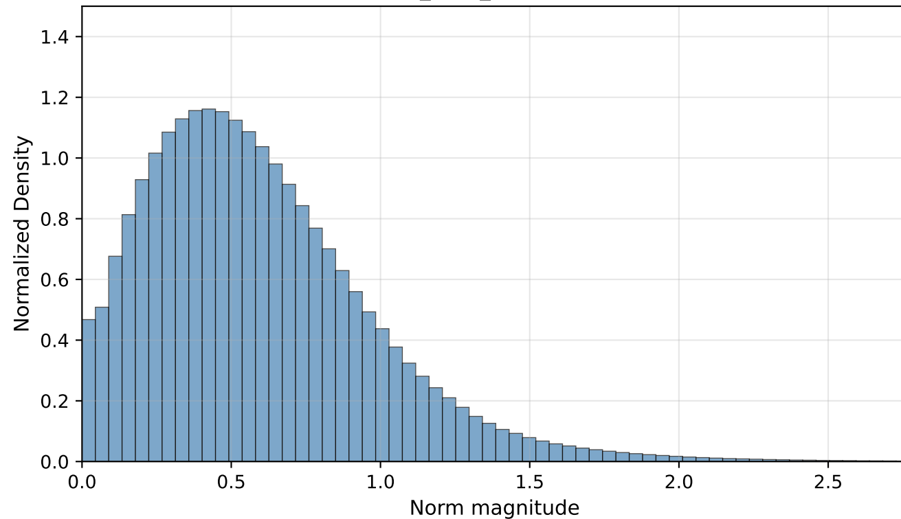
fourier_relu_16 + Normbn
