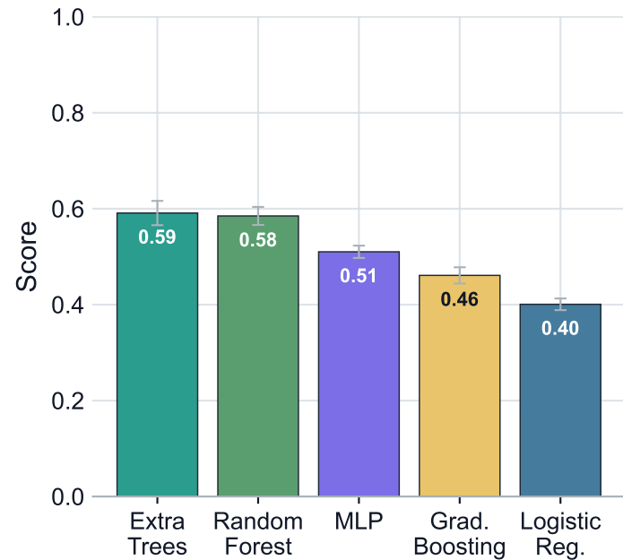
Macro F1
