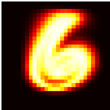
\hat{\Sigma}_6 (diag.)
