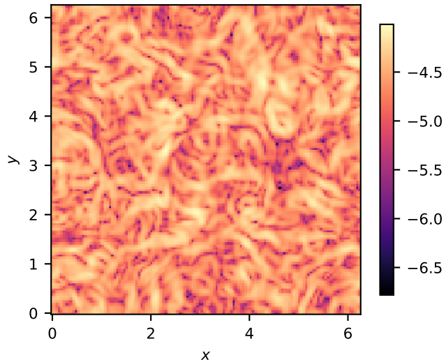
\log_{10} |u_{PINN} - u_{exact}|
