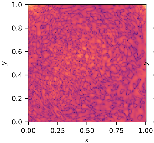
row F, hard lid: \log_{10} |\nabla \cdot u|
