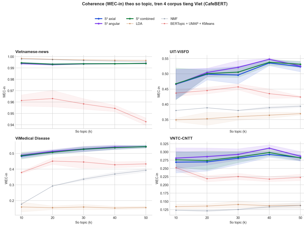
Figure 2: WEC-in (coherence) theo số trục/chủ đề, trên 4 corpus tiếng Việt \times 6 mô hình (CafeBERT). Số liệu và hình của nhóm, từ 480 lần chạy thật trong benchmark/cafebert_full/.
