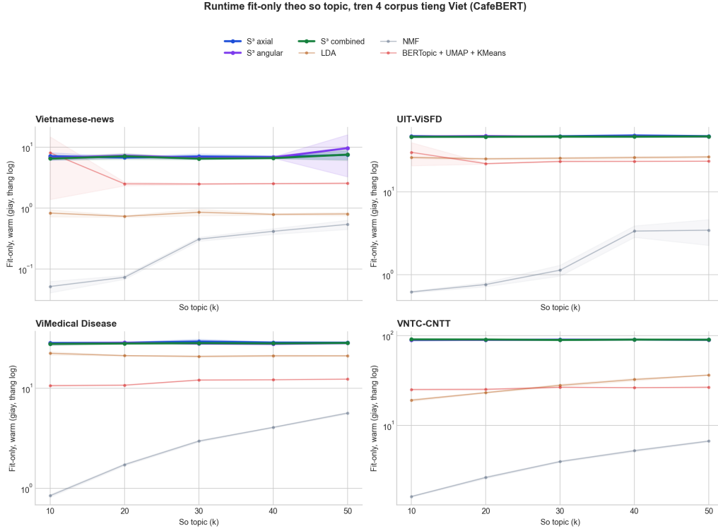
Figure 3: Thời gian fit-only (trục tung, thang log, giây) theo số trục/chủ đề. S^3 là nhóm chậm nhất trong sáu mô hình được so sánh.
