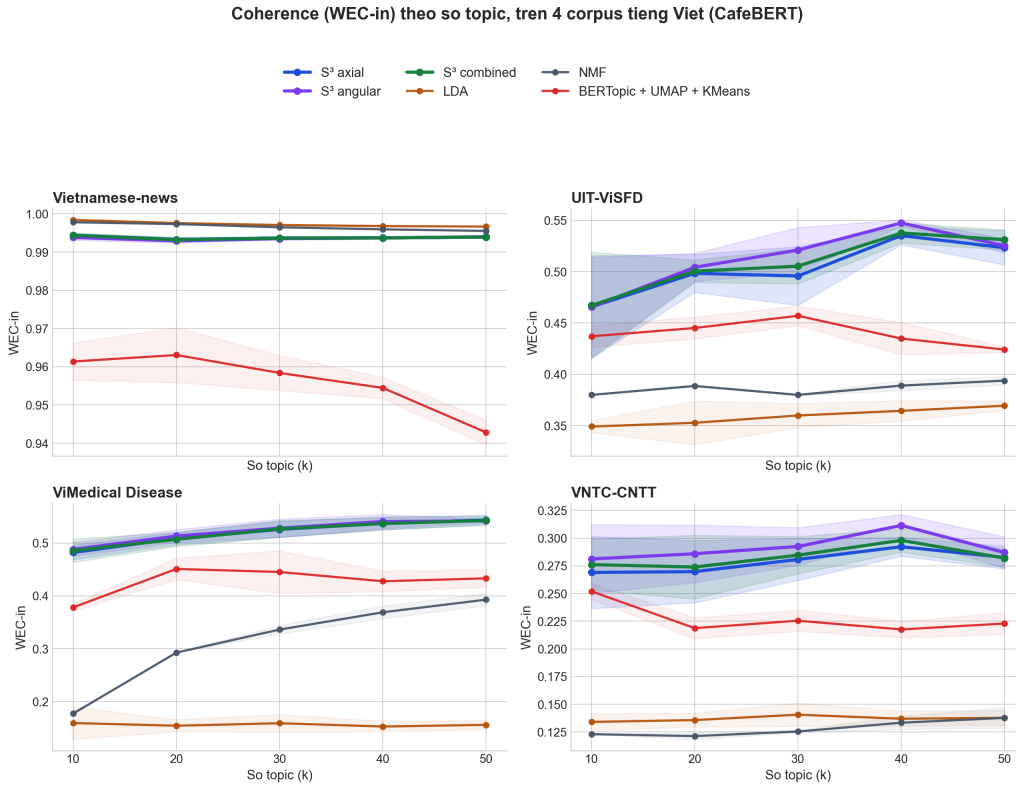
Figure 2: WEC-in (coherence) theo số trục/chủ đề, trên 4 corpus tiếng Việt \times 6 mô hình (CafeBERT). Số liệu và hình của nhóm, từ 480 lần chạy thật trong benchmark/cafesbert_full/.
