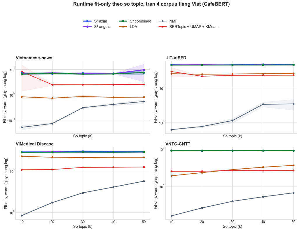
Figure 3: Thời gian fit-only (trục tung, thang log, giây) theo số trục/chủ đề. S^3 là nhóm chậm nhất trong sáu mô hình được so sánh.
