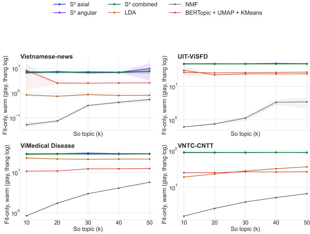
Figure 4: Thời gian fit-only (trục tung, thang log, giây) theo số trục/chủ đề. S³ là nhóm chậm nhất trong sáu mô hình được so sánh.
