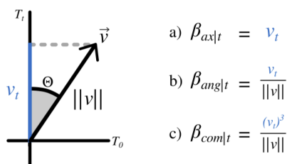
Figure 1: Trực giác hình học của ba công thức chấm điểm quan trọng từ. Tái hiện từ (Kardos et al., 2025).
