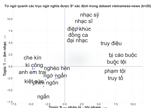
Figure 2: Concept Compass của nhóm: hình chiếu 20.000 từ vựng lên hai trục ngữ nghĩa của một checkpoint S^3 (Vietnamese-news, k = 20 ). Cực dương mỗi trục gom đúng cụm từ khoá của chủ đề tương ứng; cực âm gom các từ ít mang tín hiệu chủ đề.
