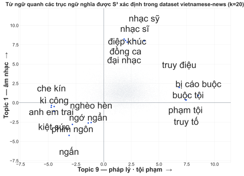
Figure 2: Concept Compass của nhóm: hình chiếu 20.000 từ vựng lên hai trục ngữ nghĩa của một checkpoint S^3 (Vietnamese-news, k = 20 ). Cực dương mỗi trục gom đúng cụm từ khoá của chủ đề tương ứng; cực âm gom các từ ít mang tín hiệu chủ đề.
