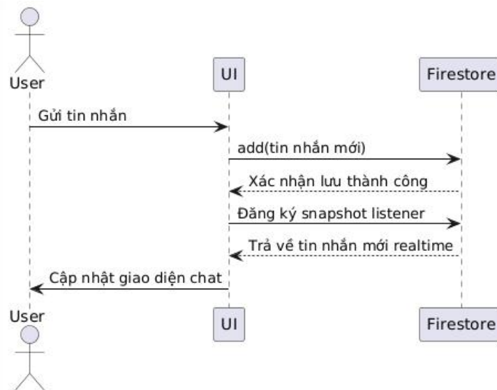
Hình 2.9. Biểu đồ tuần tự chức năng nhắn tin
