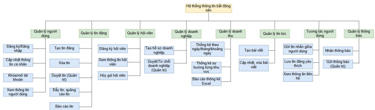
Hình 2.3. Sơ đồ phân rã chức năng
