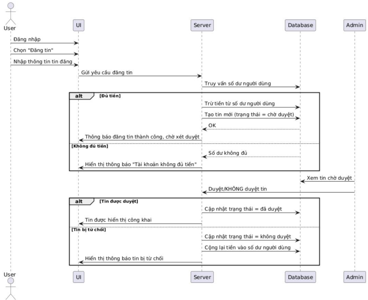
Hình 2.7. Biểu đồ tuần tự chức năng đăng tin BDS
