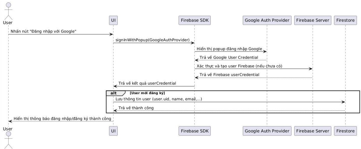
Hình 2.6. Biểu đồ tuần tự chức năng đăng ký tài khoản bằng Google
