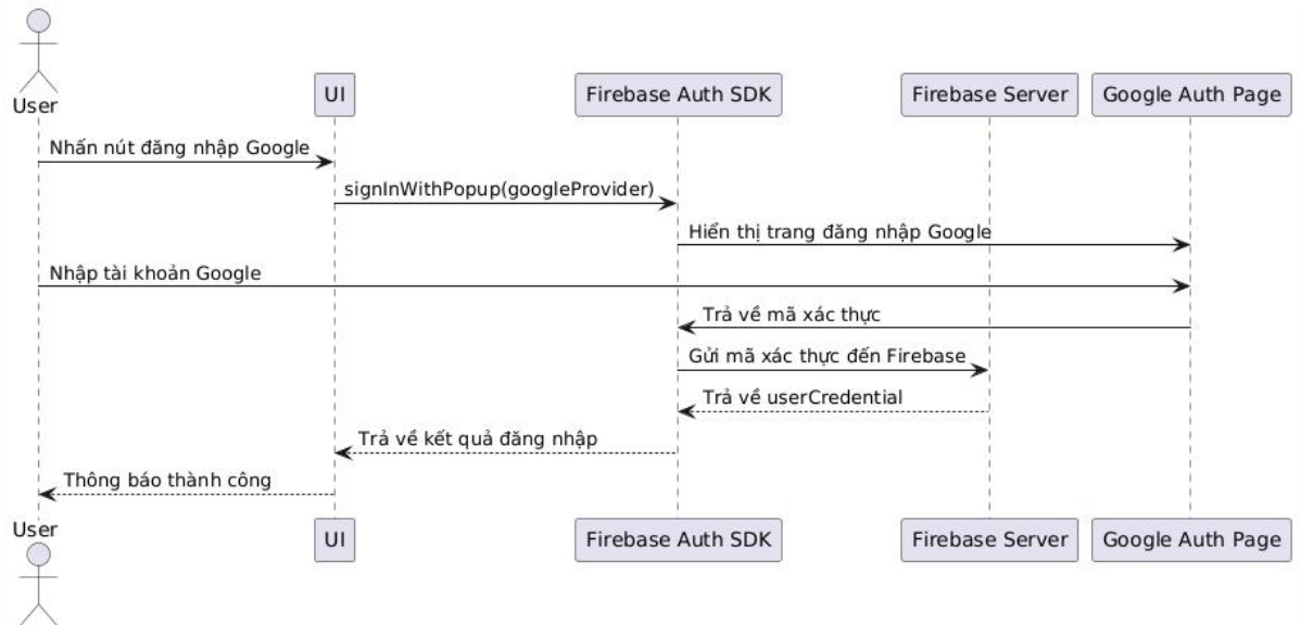
Hình 2.5. Biểu đồ tuần tự chức năng đăng nhập bằng Google
