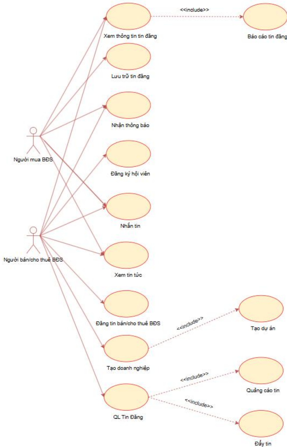
Hình 2.1. Biểu đồ use-case người mua/bán BĐS
