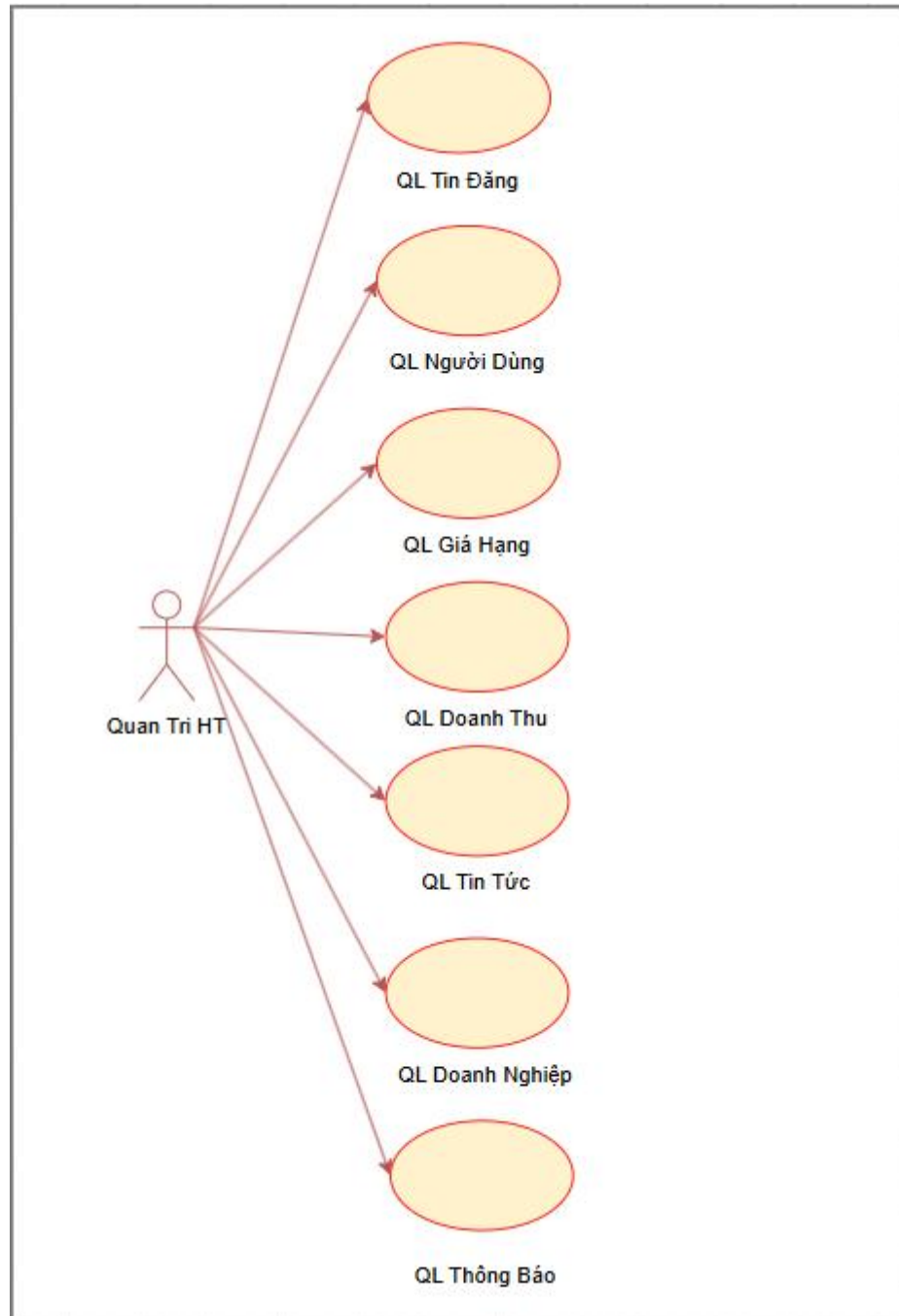
Hình 2.2. Biểu đồ use-case quản lý
