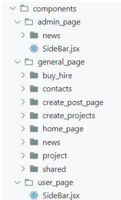
Hình 3.3. Cấu trúc thư mục components
