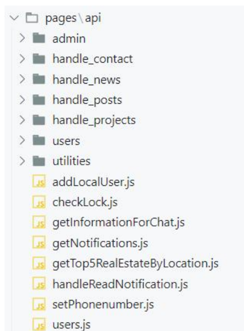
Hình 3.5. Cấu trúc thư mục pages/api/
