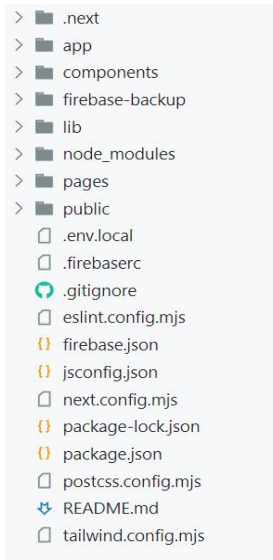
Hình 3.1. Cấu trúc thư mục dự án
