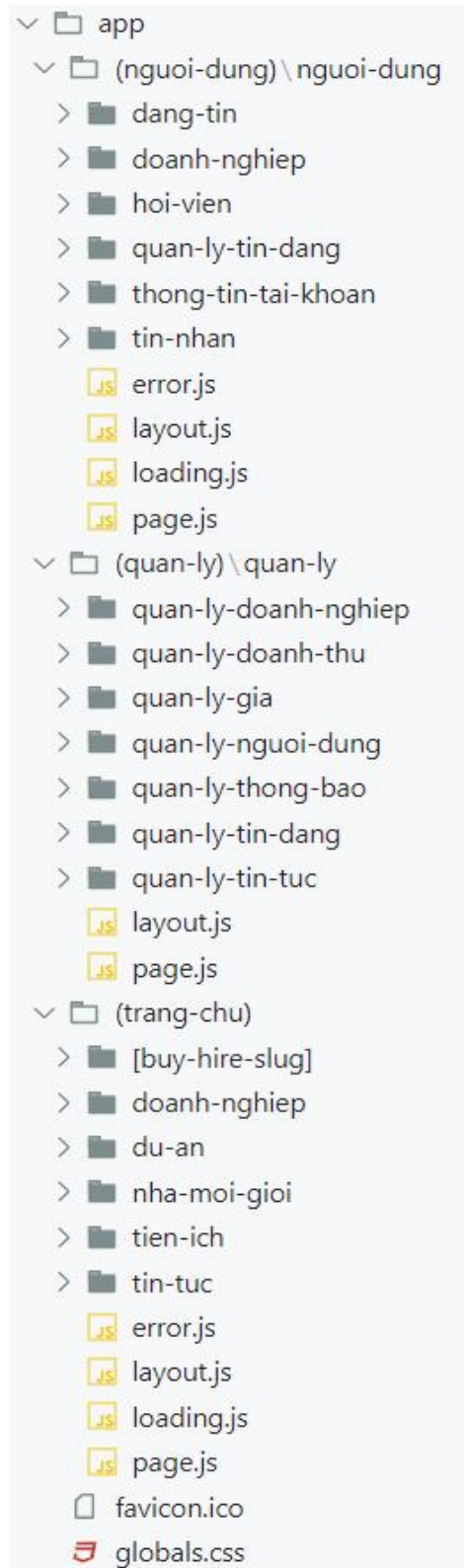
Hình 3.2. Cấu trúc thư mục app/
