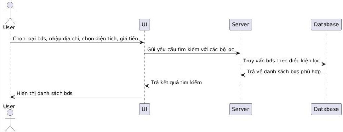
Hình 2.8. Biểu đồ tuần tự chức năng tìm kiếm tin đăng BDS
