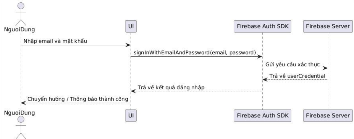
Hình 2.4. Biểu đồ tuần tự chức năng đăng nhập
