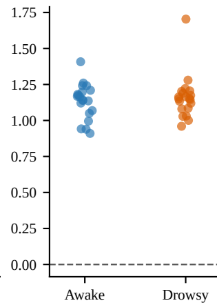
(D) Lmean
