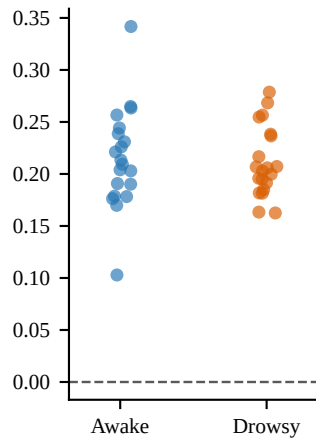
(G) LLE
