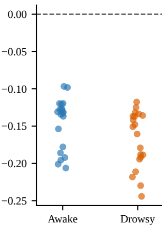
(F) TT
