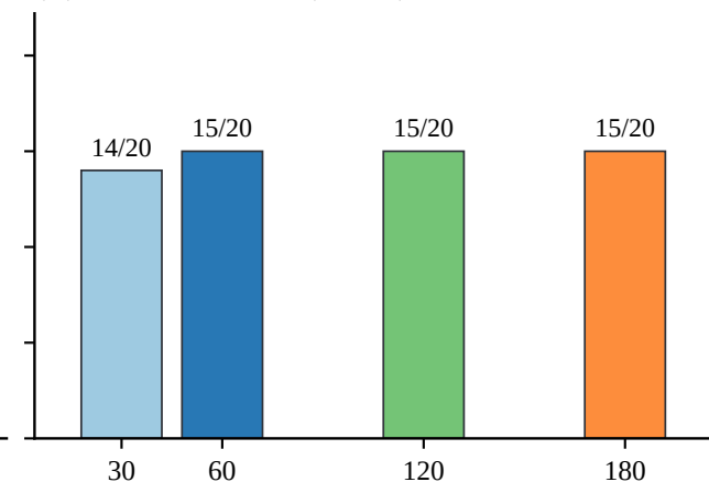
(D) LLE ( \Delta < 0 )
