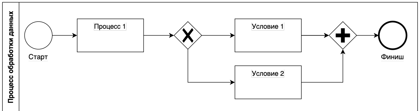
Рисунок 1. Схема алгоритма 1
