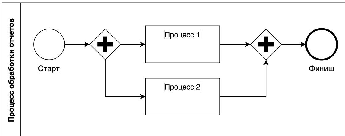
Рисунок 2. Схема алгоритма 2
