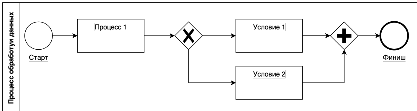
Рисунок 1. Схема алгоритма 1
