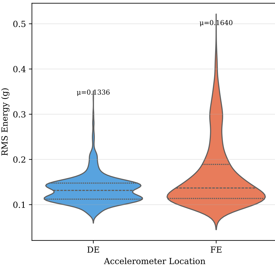
Fig. 9a: RMS Energy DE/FE attenuation: -1.8 dB
