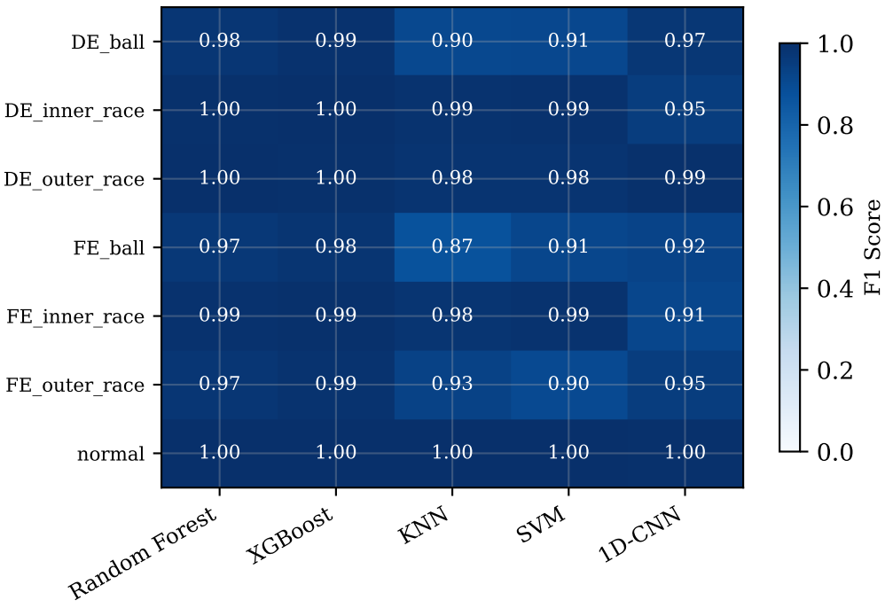
Per-Class F1 Score Heatmap
