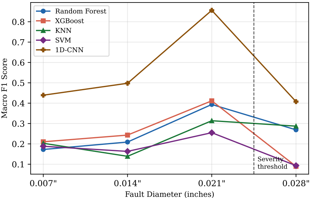
Macro F1 vs Fault Size (Hold-One-Size-Out)
