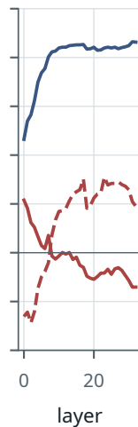
OLMo-2-7B
