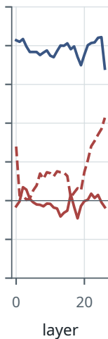
Gemma-2-2B
