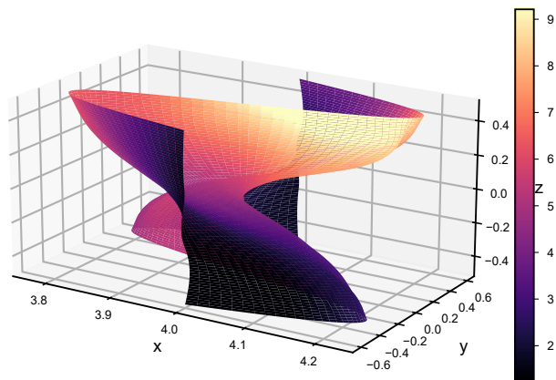
von Mises stress
