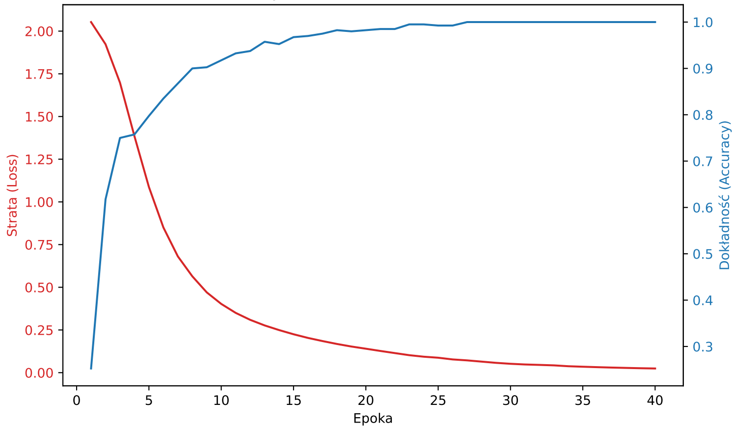
Krzywe uczenia LeNet-5 (8 klas)
