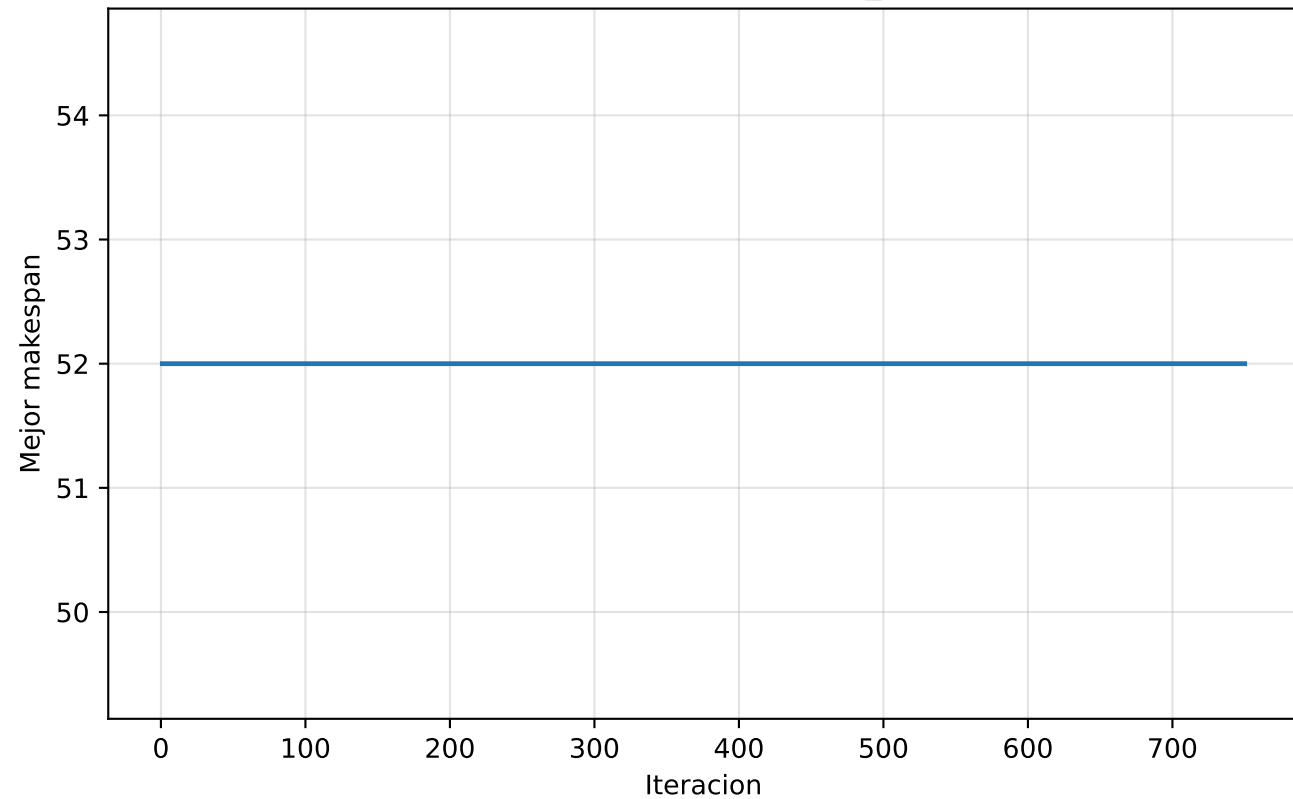
Convergencia - instancia1_bas1
