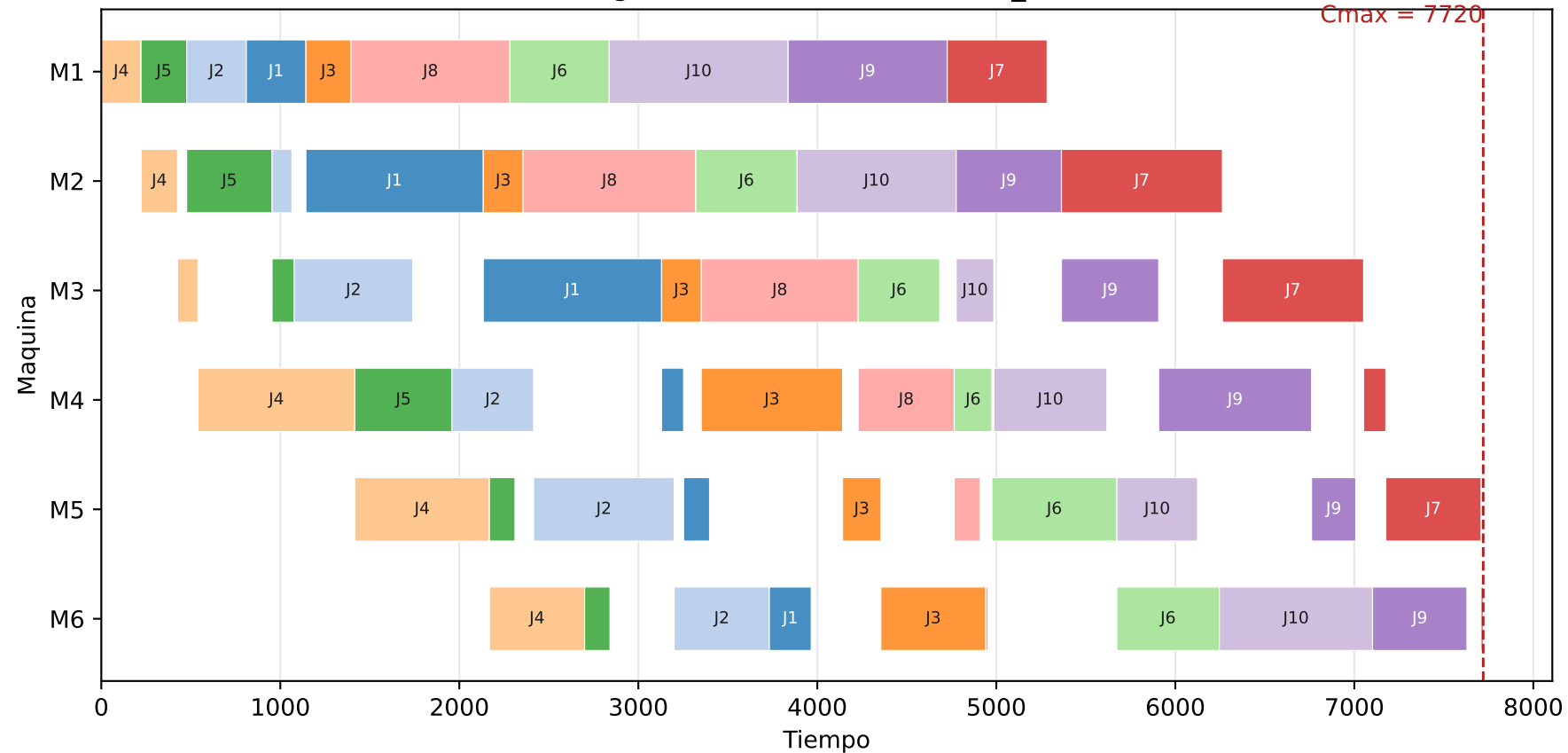
Diagrama de Gantt - instancia2_car5
