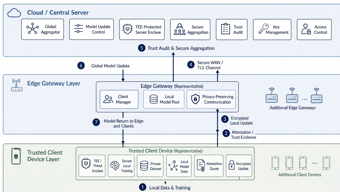
图 1: 联邦计算网络交互：基于 TEE 锚点加密的端边云协同物理架构图
