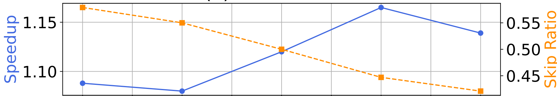
(a) LLaMa-2-13B
