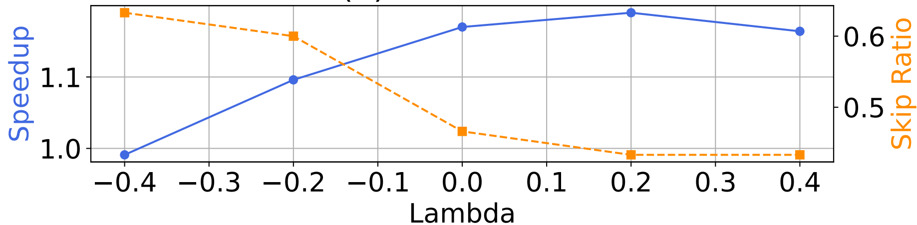
(b) LLaMa-3-8B
