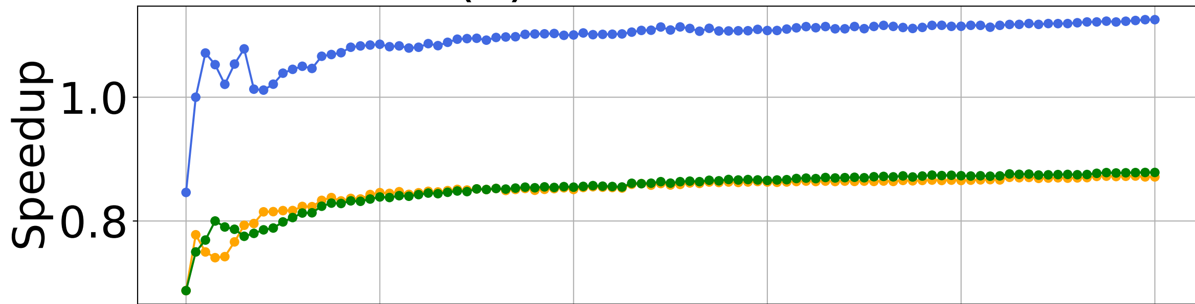
(a) LLaMa-2-13B
