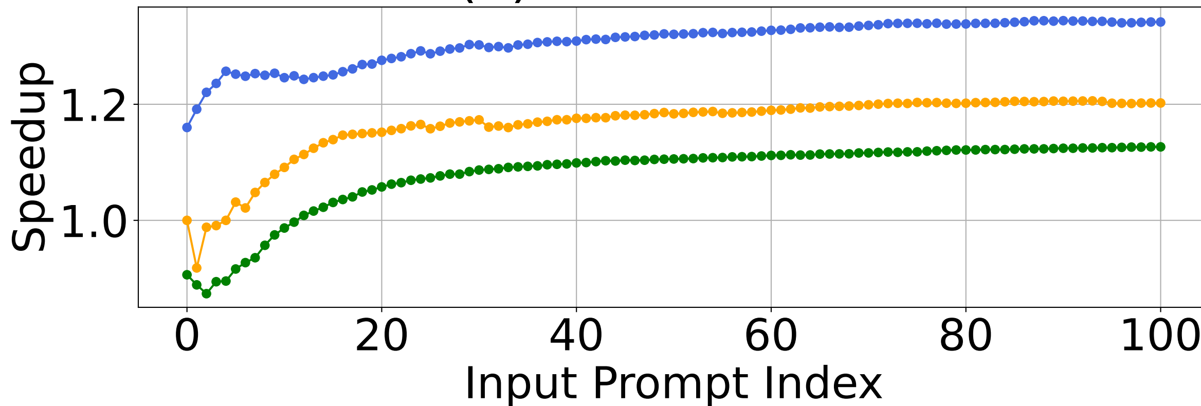
(b) LLaMa-2-70B
