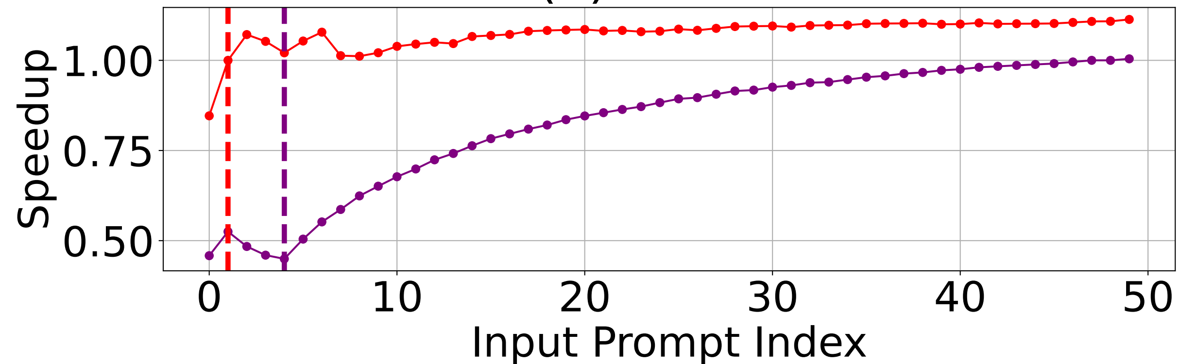
(b) GSM8K
