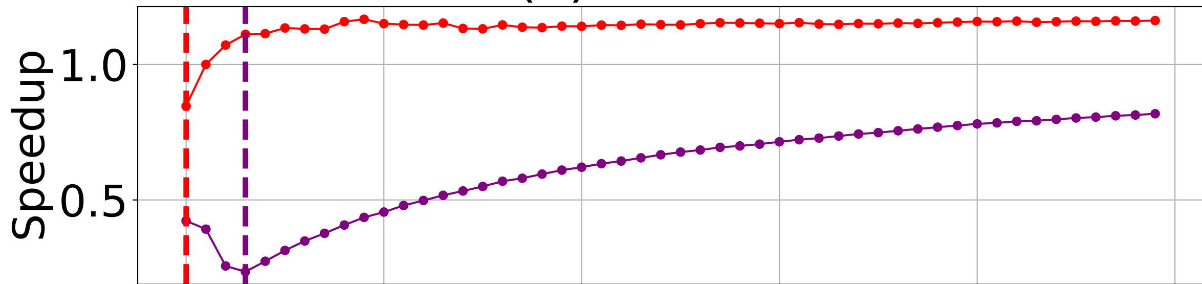
(a) CNN-DM
