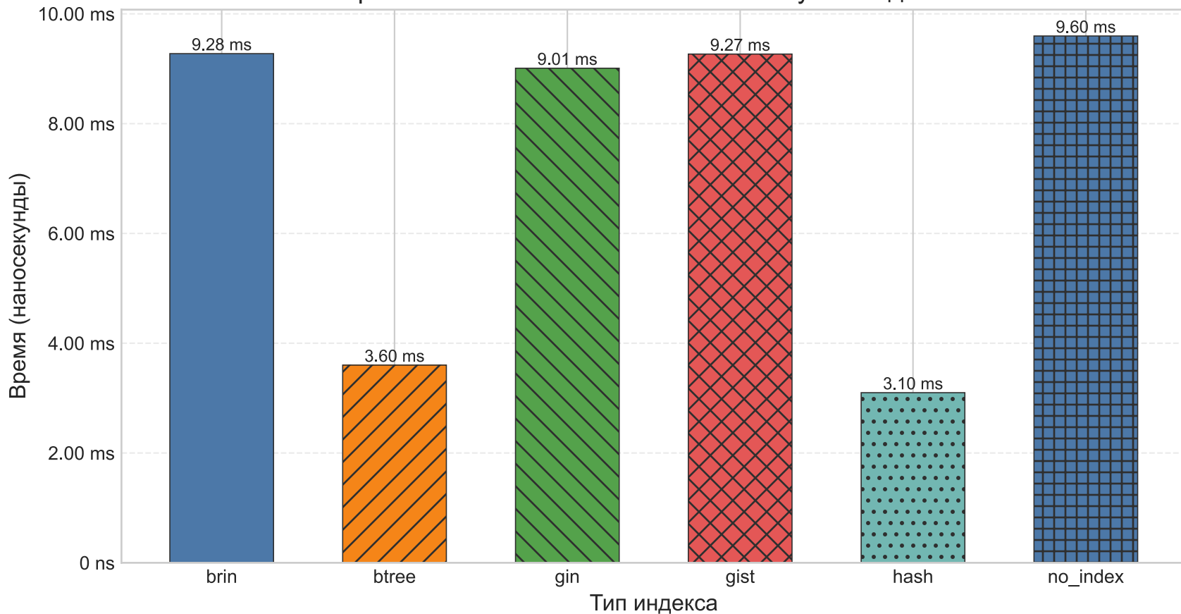
Время выполнения поиска по точному совпадению
