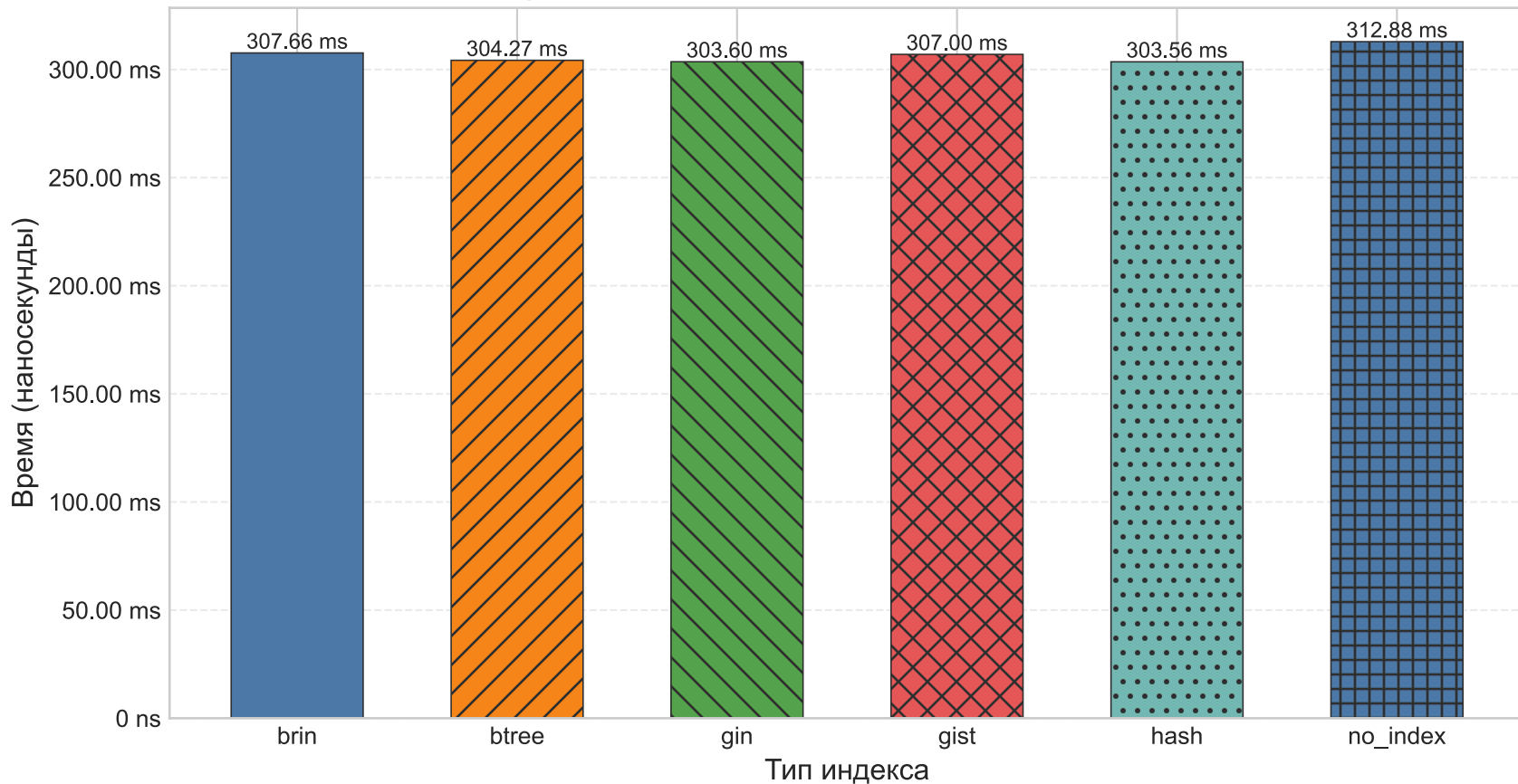
Время выполнения полнотекстового поиска
