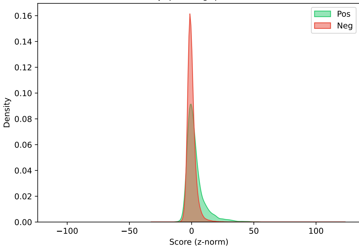
Full | sparse (gap=3.211)
