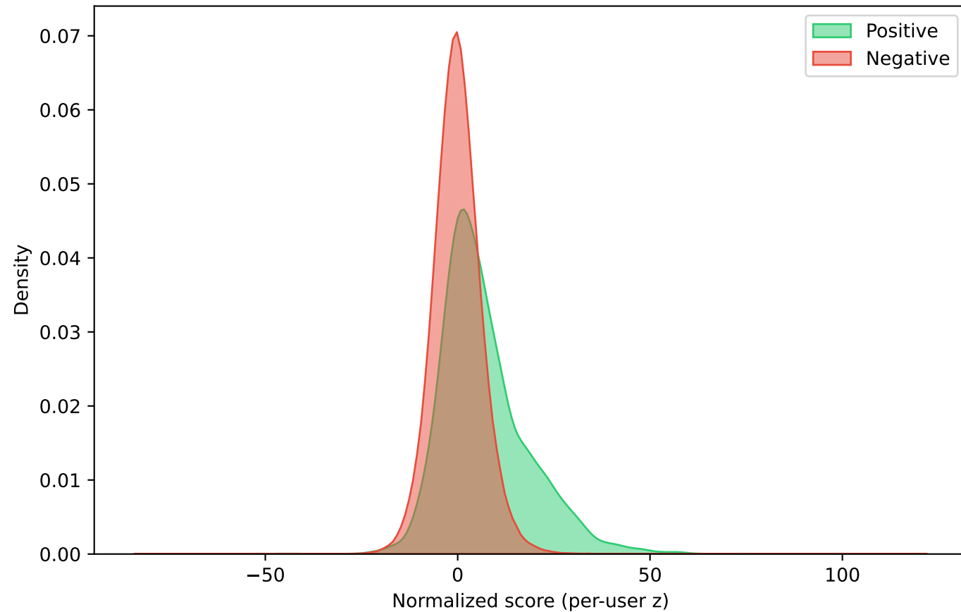
Base: gap = 6.987
