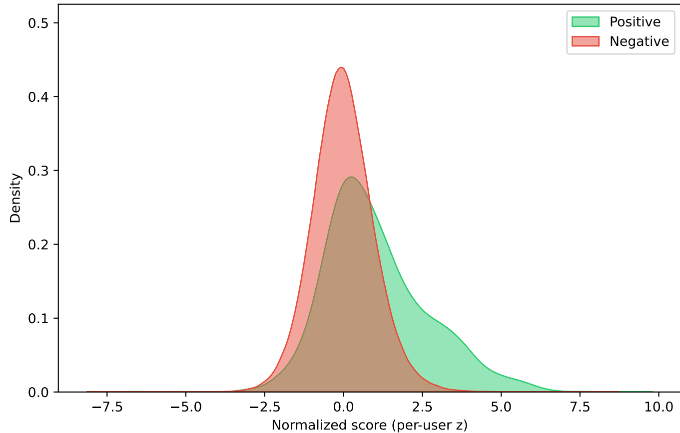
Base: gap = 1.043
