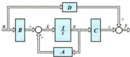
图 9-2 线性连续时间系统结构图
