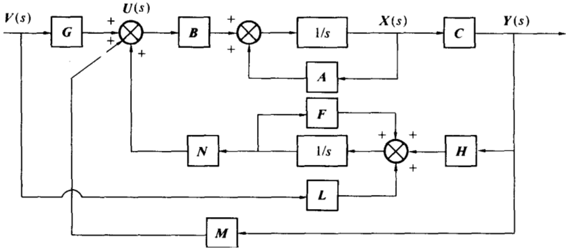
图 5: D = 0 时动态补偿器的方块图
