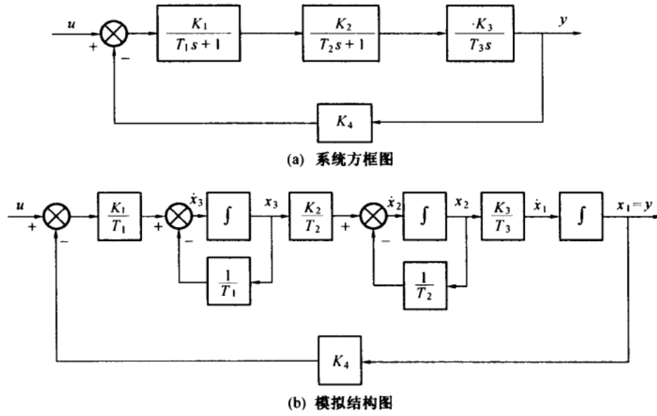
图 2: 系统模拟结构图
