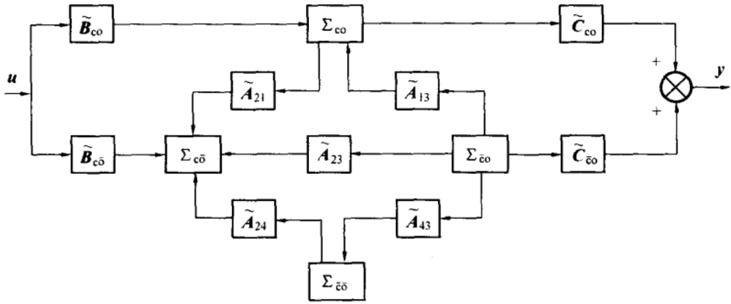
图 3: 系统结构规范分解
