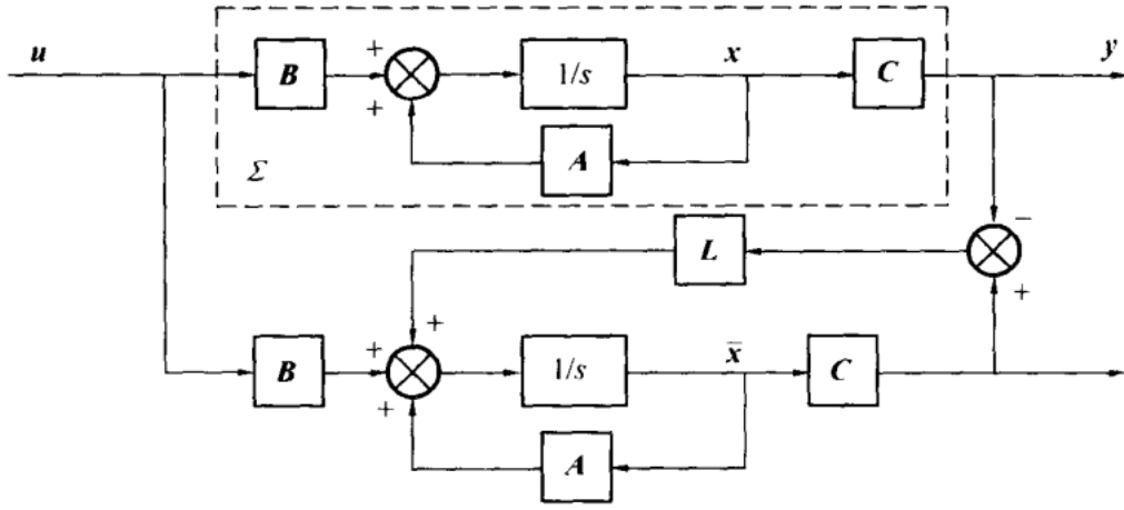
图 6: 全维观测器的结构图
