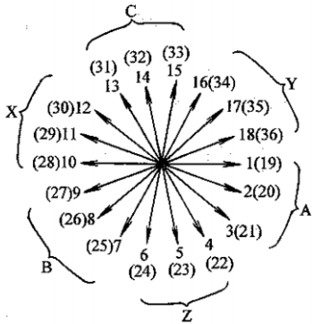
图 4.1: 三相双层绕组槽电动势星形图 ( Q = 36, 2p = 4 )
