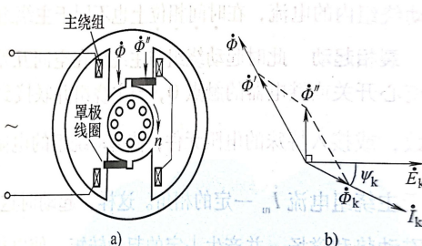
图 5.11: 罩极式单相感应电动机
