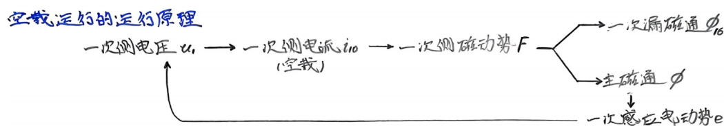
图 2.2: 变压器空载运行的基本原理
