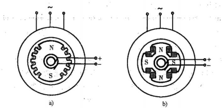
图 6-1 旋转磁极式同步电机的类型 a) 隐极式 b) 凸极式
